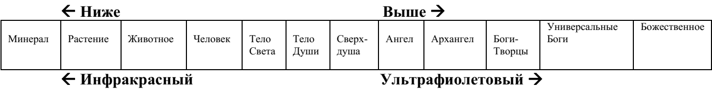
Рисунок 9.1 Плотности как функция спектра света
